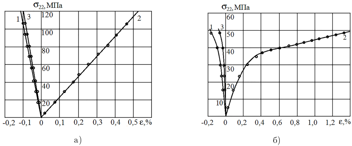
Рис. 2: Диаграммы деформирования вдоль оси x_2 : а) растяжение; б) сжатие; 1, 3 – поперечные деформации \varepsilon_{11} и \varepsilon_{33} ; 2 – продольная деформация \varepsilon_{22} ; \circ – экспериментальные данные; ——— – нелинейные аппроксимации
