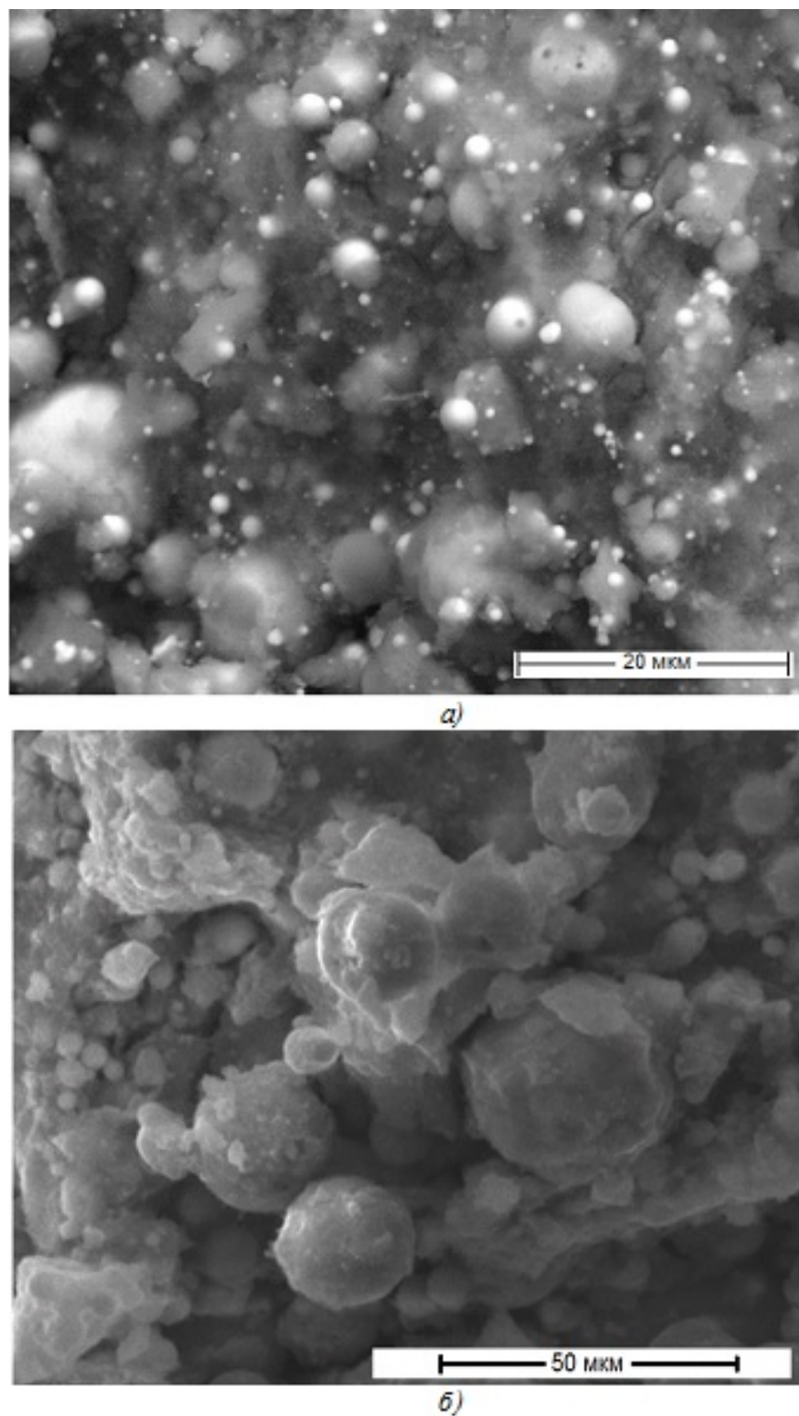
Рис. 6: Микрофотография частиц электроэрозионной шихты, полученной: а) в воде дистиллированной; б) керосине осветительном (растровый микроскоп QUANTA 600 FEG)
