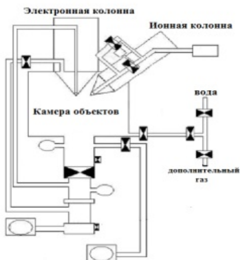
Принципиальная схема процесса исследования шихты
