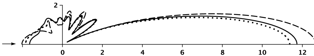
Рис. 1: Диаграммы направленности
