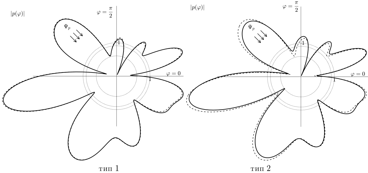
Рис. 5: Влияние анизотропии
