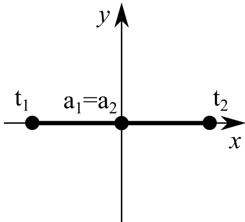
Рис. 2: Случай r = 0
