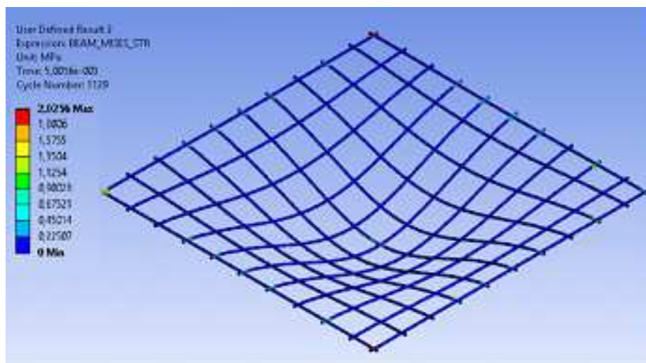
Рис. 10: Схема деформированной арматуры в плите
