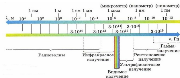
Рис. 5: Шкала электромагнитных волн [11].
