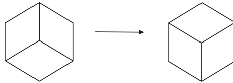
Рис. 1. Пример перекладывающегося разбиения.
