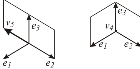
Рис. 6. Возможные соседи слева ромба \mathbb{R}_i^N .
