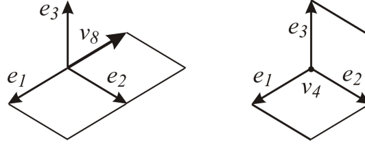
Рис. 12. Возможные соседи справа и сверху ромба \mathbb{B}_i^N .
