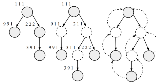
Рис. 1: Исходное и промежуточные представления (слева направо): дерево процессов T , некоторый его граф восстановления G(T) и дополненный зависимостями (мульти)граф G(T) \cup DEP(T) . Числа при вершинах – атрибуты-идентификаторы процесса P , группы G и сессии S соответственно. Корневой процесс всегда имеет идентификаторы “1,1,1”.
