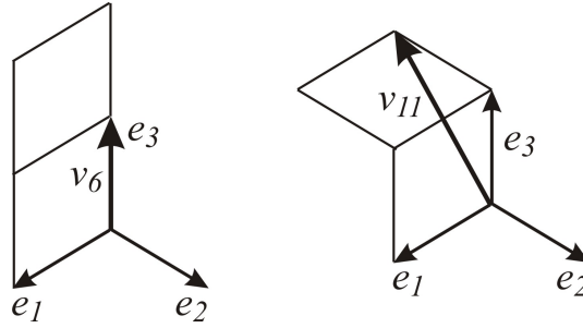
Рис. 11. Возможные соседи сверху ромба \mathbb{G}_i^N .
