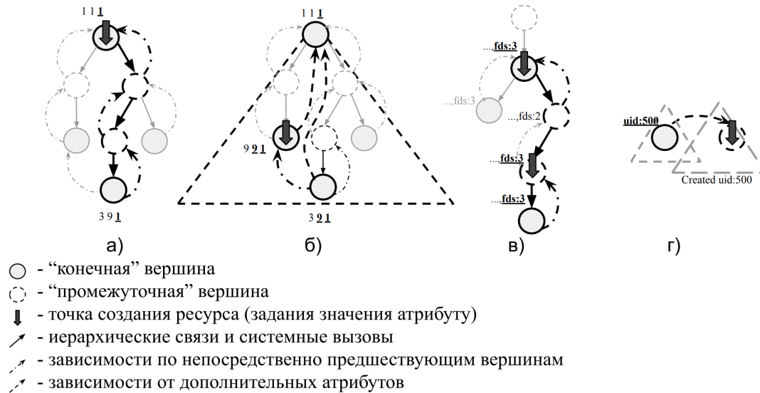
Рис. 3: Типы атрибутивных зависимостей: а) строго наследуемые; б) выставляемые в подобласти; в) нестрого наследуемые; г) свободные.
